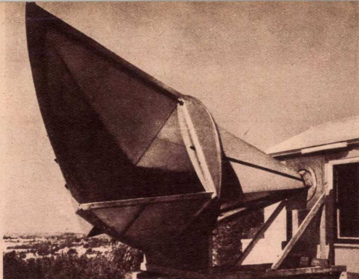
Az Echo-kísérletekhez használt tölcsérantenna. Önműködően nyomon követi az Echo I-et és felveszi a róla visszaverődött rádióhullámokat
